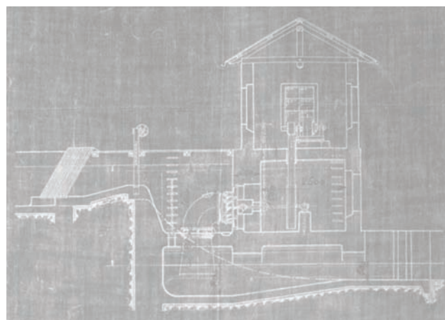
Plan hidrocentrale
